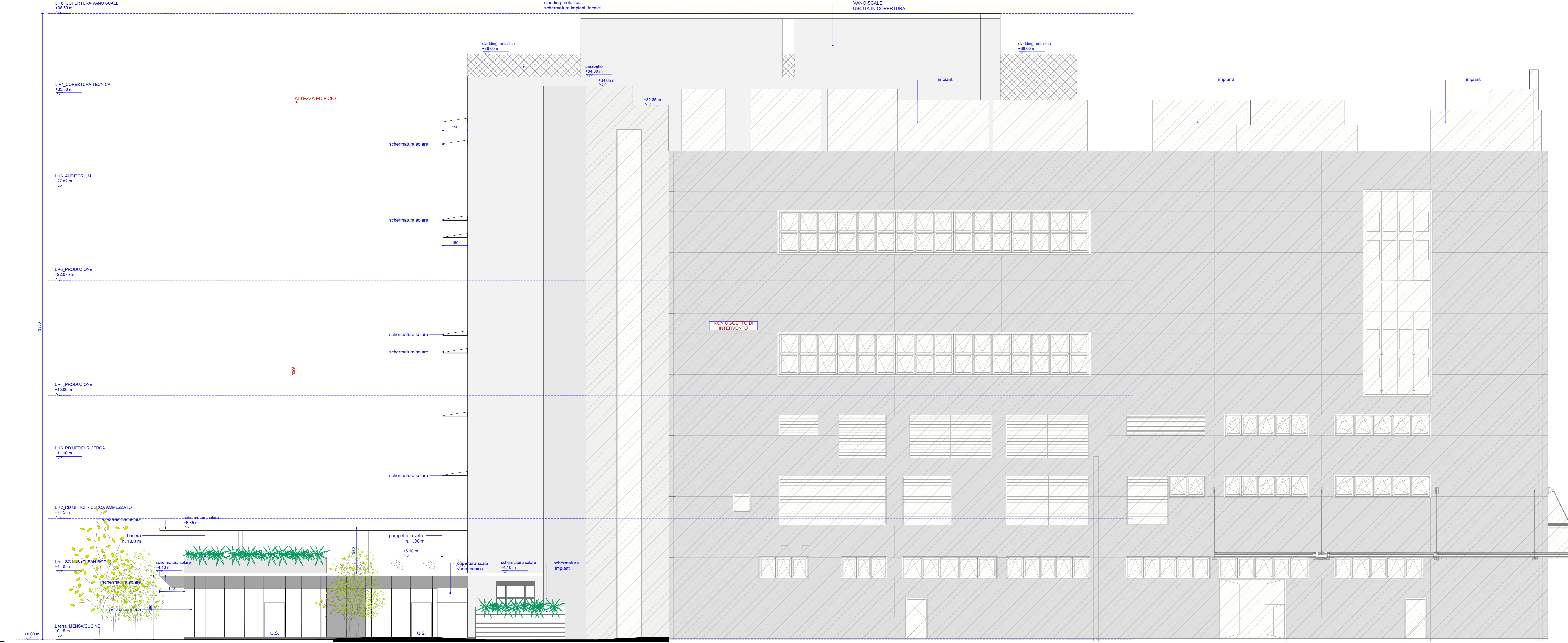
P4_PROSPETTO NORD, scala 1:100
