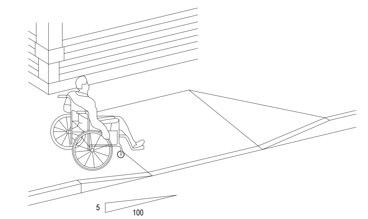
PENDENZA RAMPE NEI PERCORSI ESTERNI SCALA 1:20
