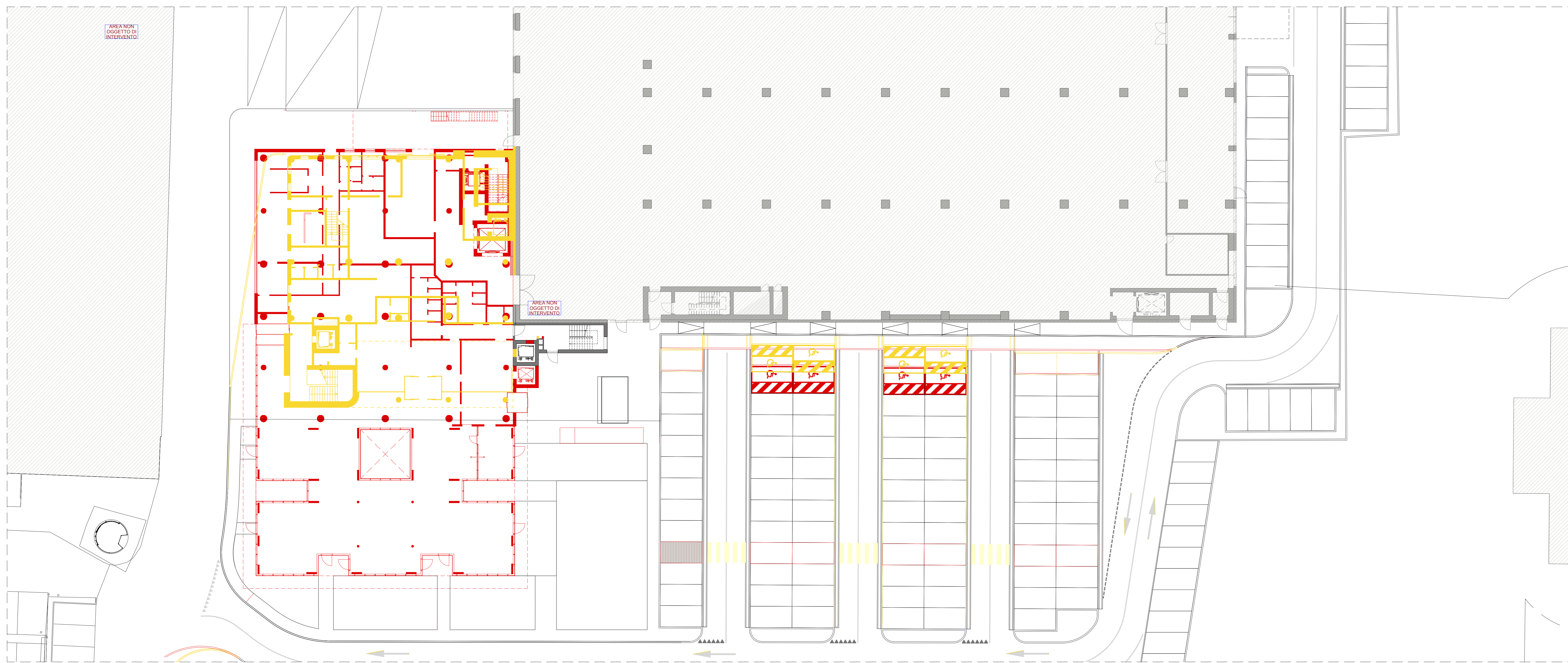
PIANTA PIANO TERRA, +0.15, MENSA-CUCINA
