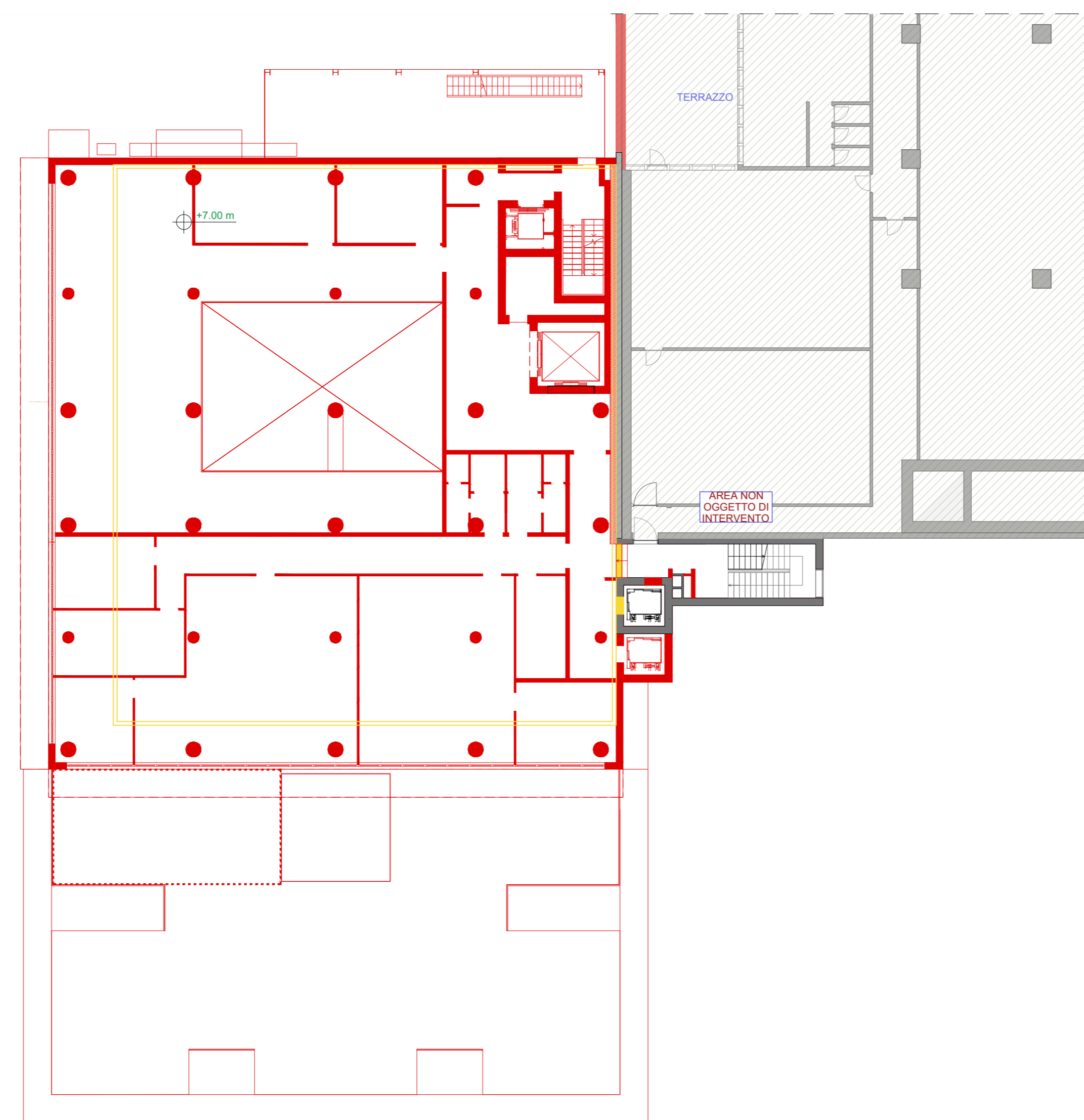
PIANTA PIANO SECONDO, +7.45, RD UFFICI RICERCA AMMEZZATO
